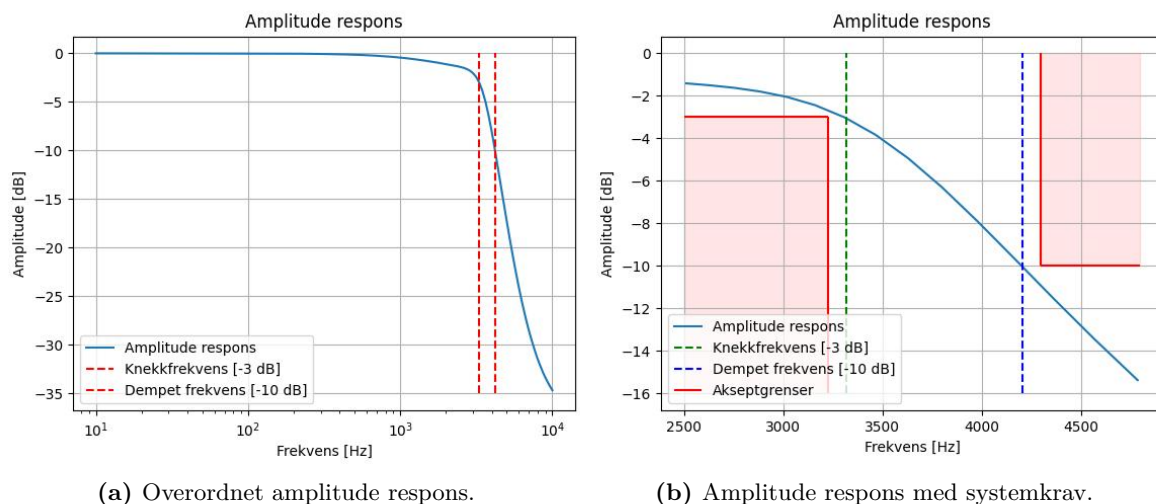
Figur 7: Amplitude respons til systemet
